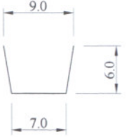
Circ Groove (2:1 scale)
