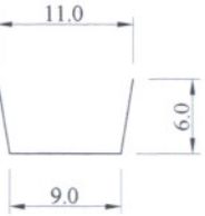
Lateral Groove (2:1 scale)
